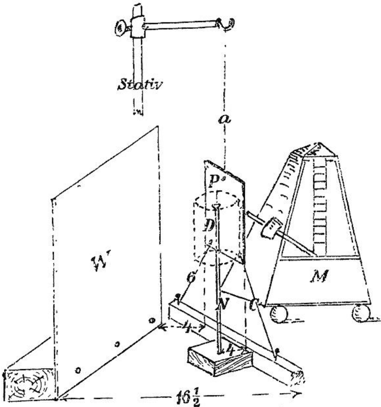
Fig. 27 b. Ansicht.
